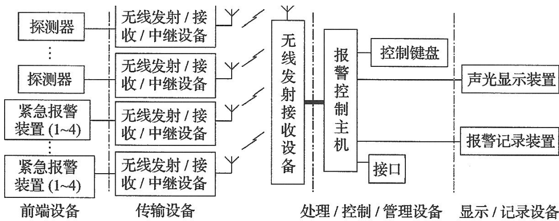
图 4.0.2-3 无线制模式
