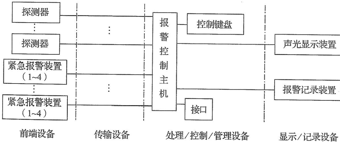
图 4.0.2-1 分线制模式
