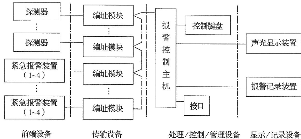
图 4.0.2-2 总线制模式
