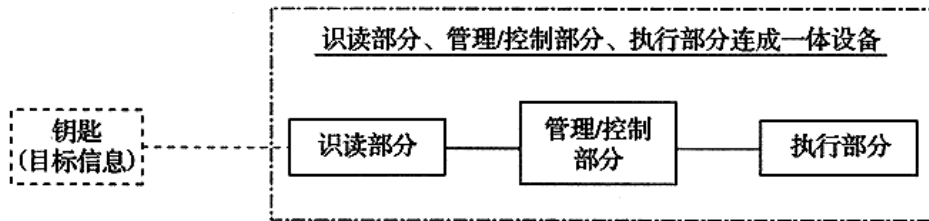
图 4.0.2-1 一体型产品组成
