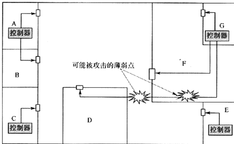
图 8 电控锁连线的布设对安全的影响
