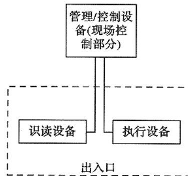
图 4.0.4-1 单出入口控制设备型组成
