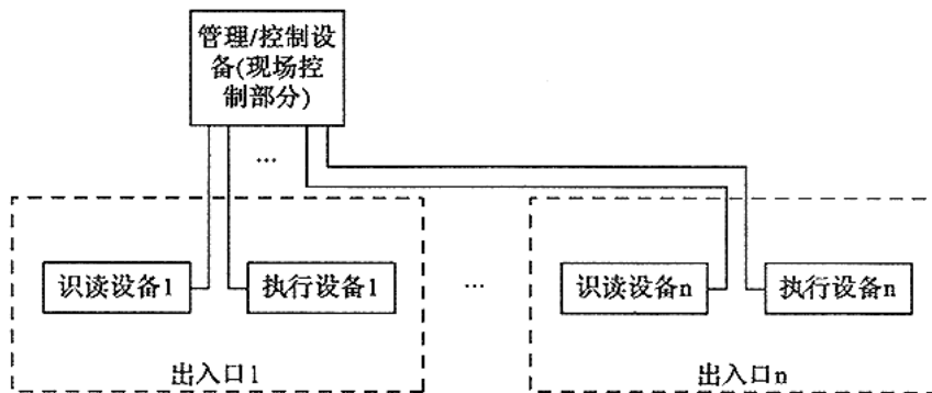
图 4.0.4-2 多出入口控制设备型组成
