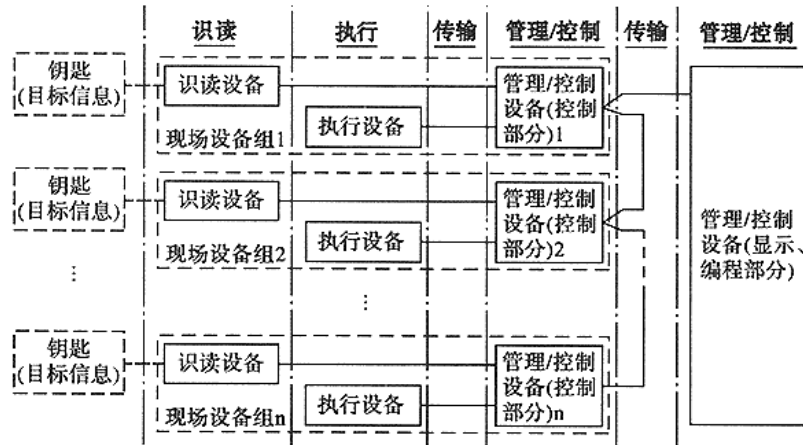
图 4.0.5-1 总线制系统组成
