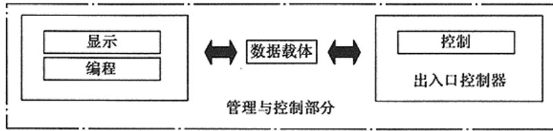
图 4.0.3-3 数据载体传输控制型组成
